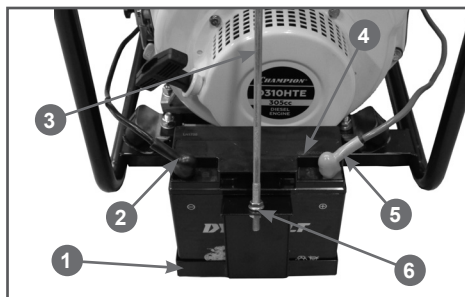
Рис. 5 Установка аккумулятора
