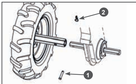
Рис. 6 Установка колес
