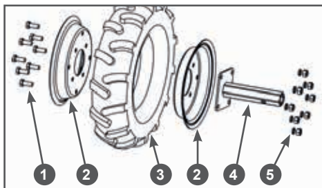
Рис. 5 Сборка колеса
