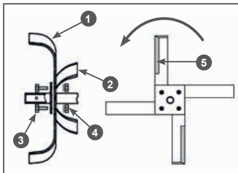
Рис.2 Сборка правой фрезы
