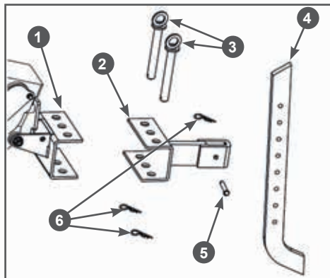
Рис. 3 Установка сошника
